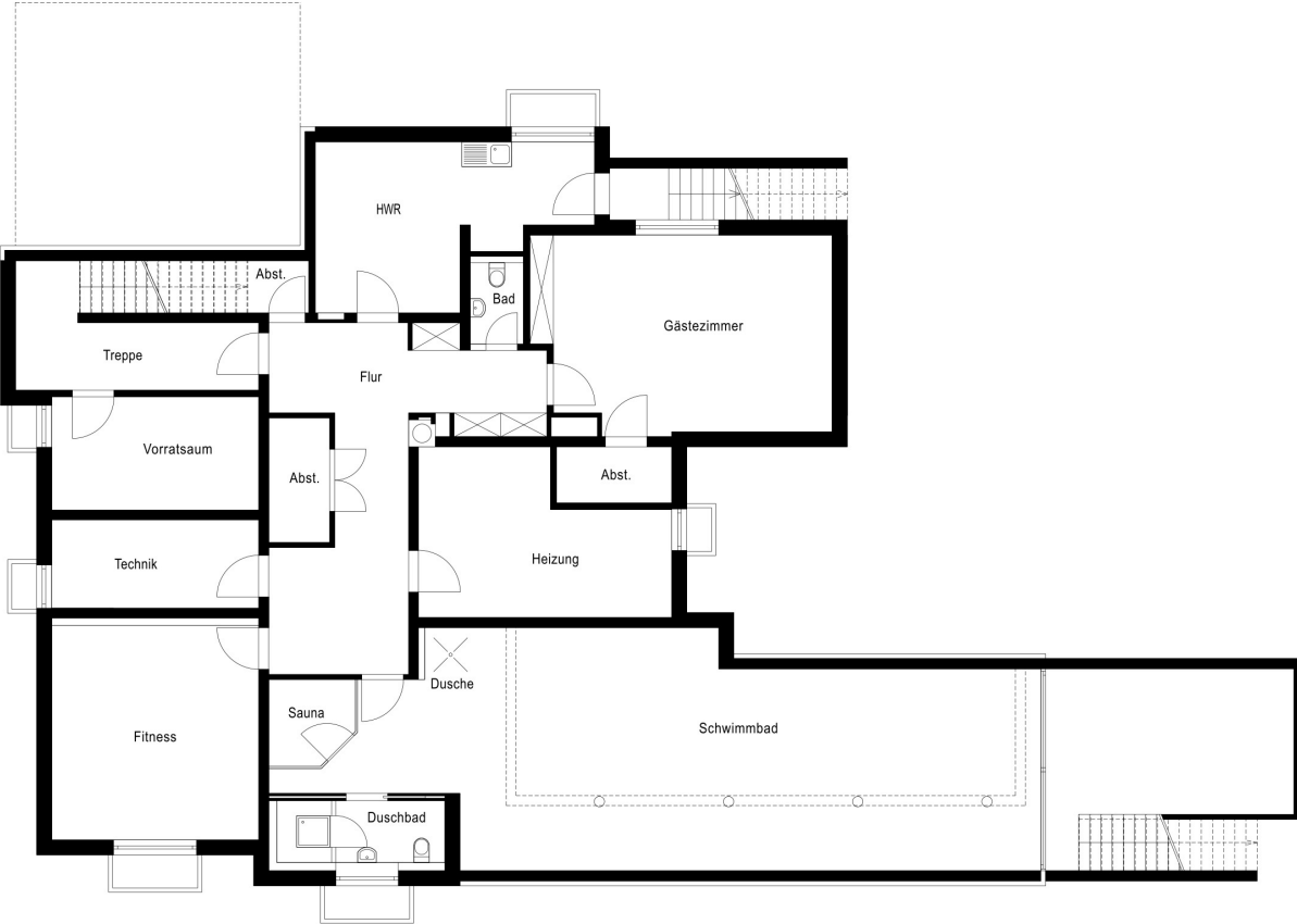
Untergeschoss
