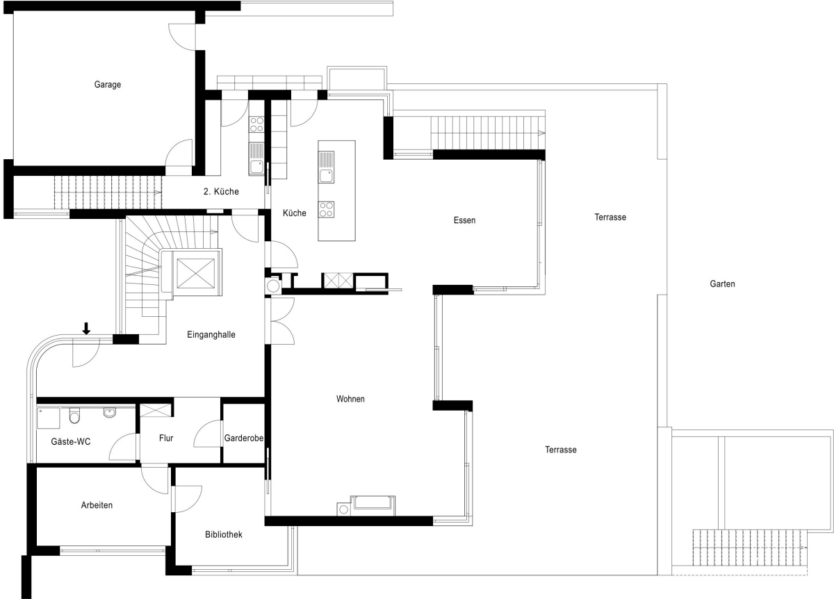
Erdgeschoss
